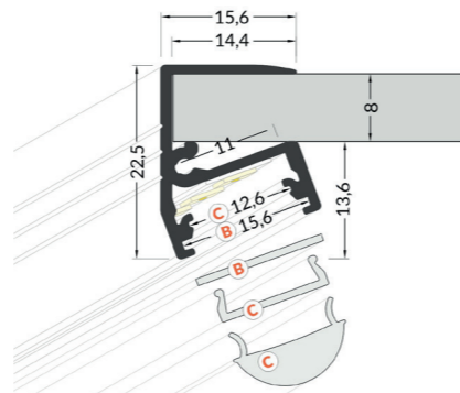
Terminaison profilé LED bord-10 Ref T98T503G
