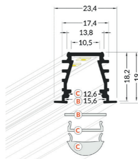
Terminaison profilé LED profond-10 - Ref T98T203G
