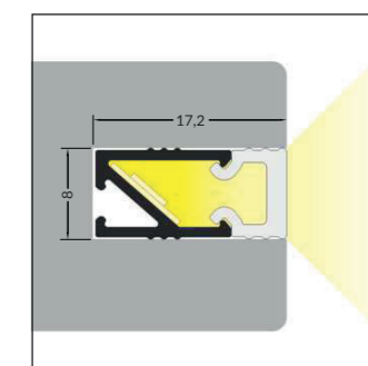
Terminaison profilé LED href-8 Gris : Ref T98T202G
