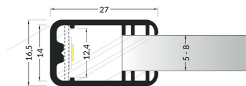
Terminaison profilé LED Glass Line-12 Ref T98T502G
