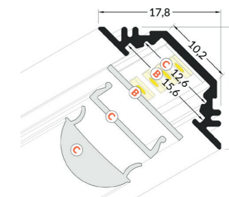
Terminaison profilé LED angle 45°-10 Ref T98T301G
