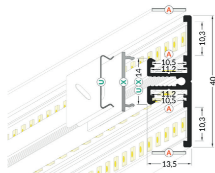
Terminaison profilé LED arrière-10 - Ref T98T402G
