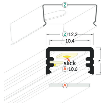
Terminaison profilé LED fin-8 - Ref T98T101G
