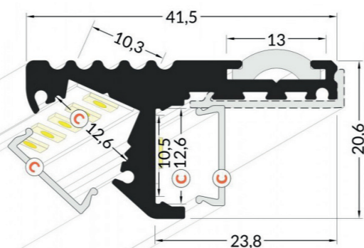
Terminaison profilé LED marche-10 - Ref T98T403G
