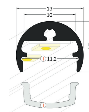
Support Double 100mm avec cache profilé LED tube-8 - Ref T98S0013
